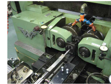
通过滚丝模进行的冷轧加工 Rolling process by Rolling dies
