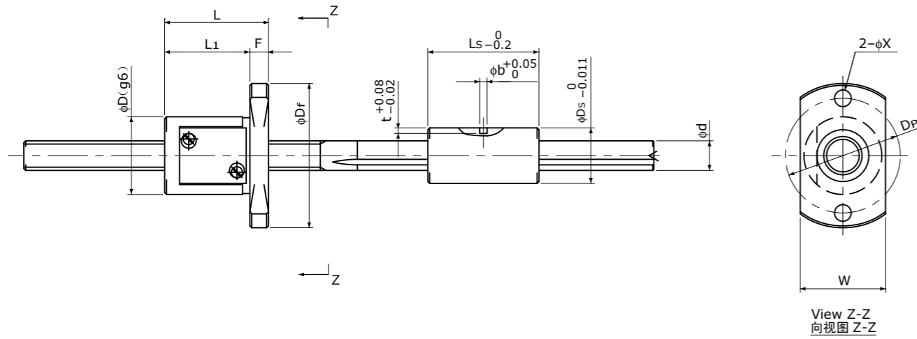
Type-1 : Return-plate type (Ball Screw Nut) 复式回路板循环方式 (滚珠丝杠螺母)
