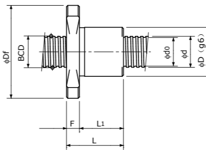
Type-2:Internal-deflector type or End-deflector type 陀螺式循环方式或偏转器式循环方式
